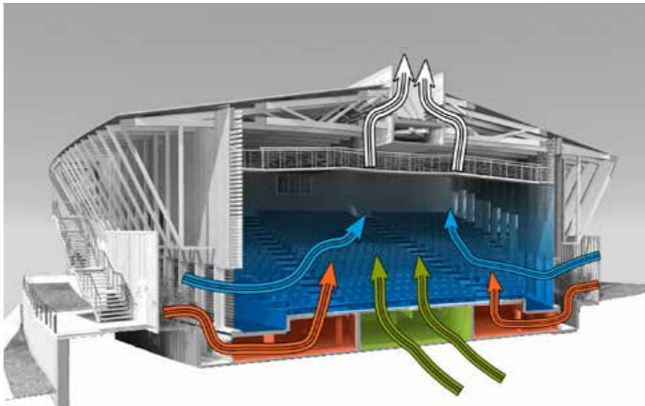
Figure 44 - Mécanisme de ventilation naturelle avec puits dépressionnaire
