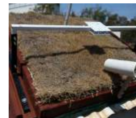
Figure 20 – Test de gazon en toiture
